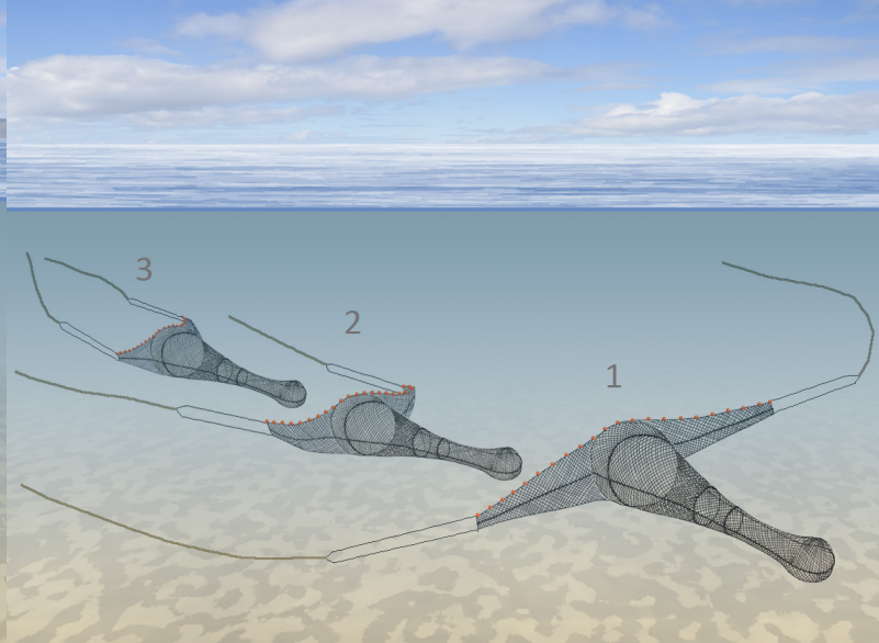
Scottish seine
