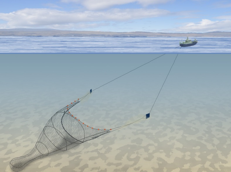
Demersal trawl
